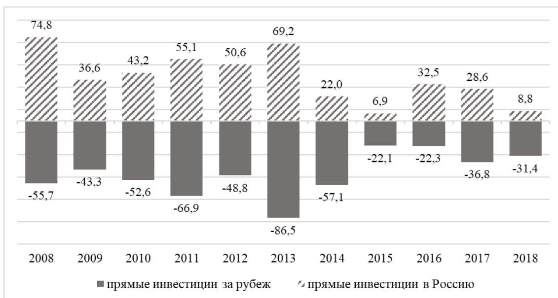
Рис. 1. Прямые инвестиции в Россию и за рубеж с 2008 по 2018 гг., млрд долларов США [4]
