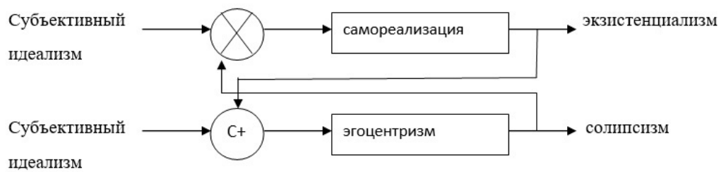
Рис. 2. Схема компенсационного гомеостата противоречия «самореализация-эгоцентризм» с обратной связью константой
